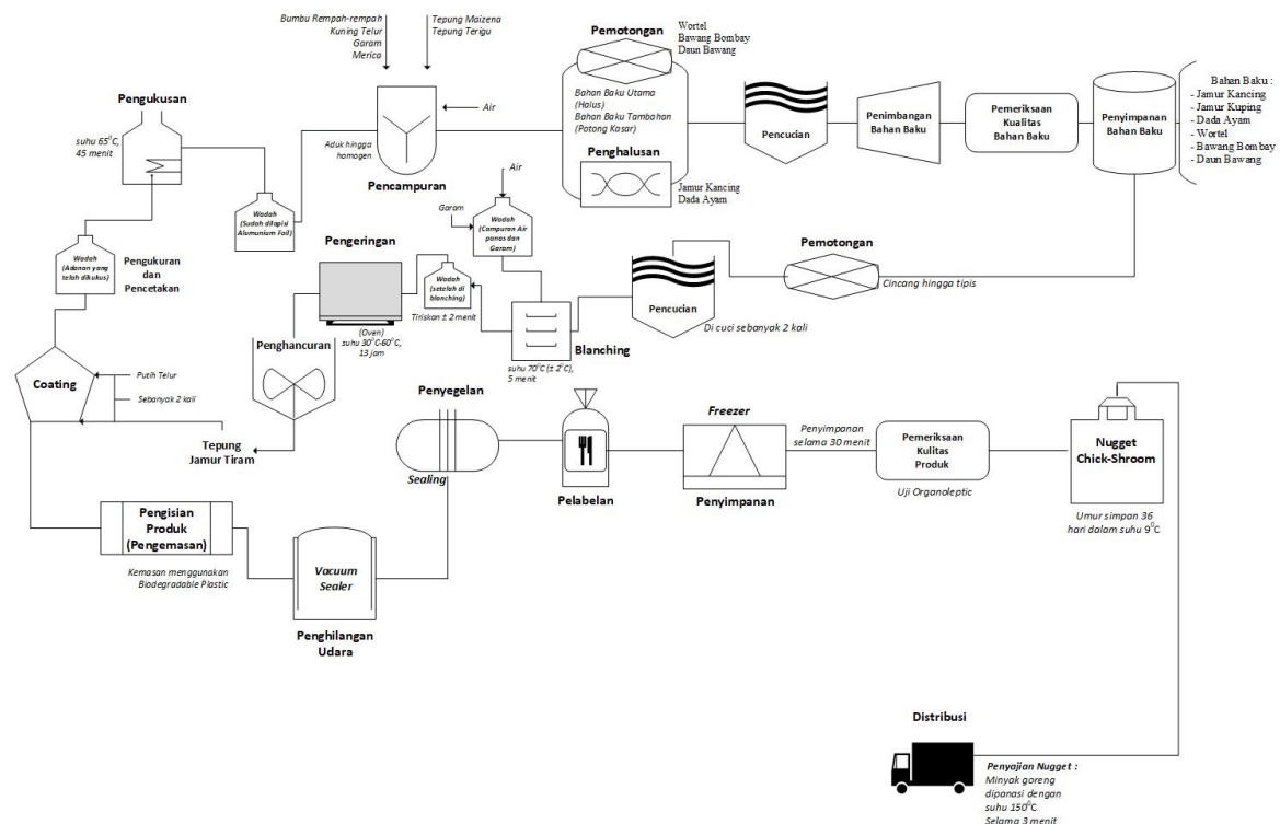
Gambar 1. Diagram Alir Proses Pembuatan Nugget Chick-Shroom
